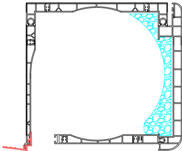
AISLANTE CURVO + BITUMINOSO
